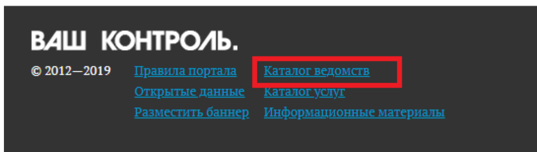
Рисунок 1. Каталог ведомств
