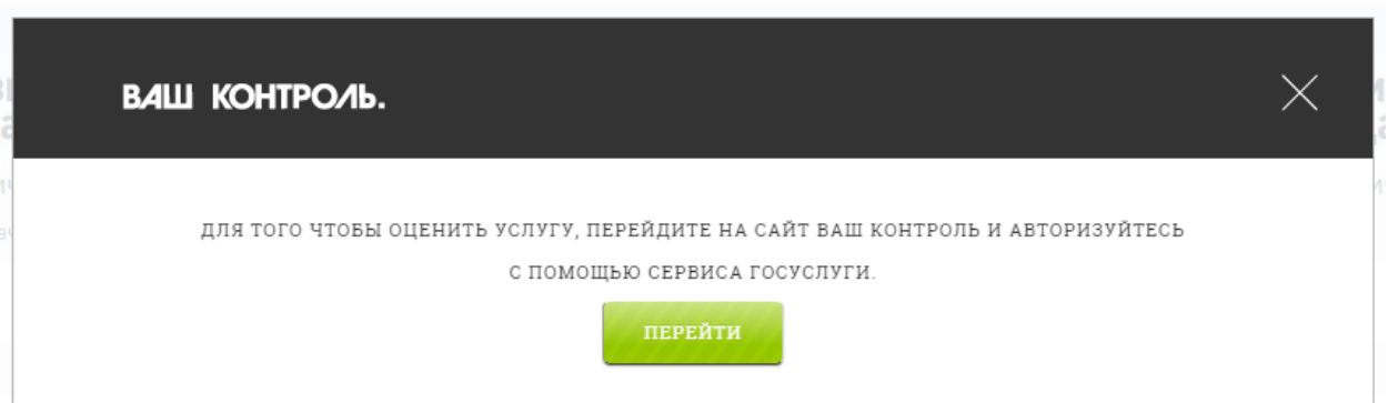
Рисунок 8. Окно виджета
